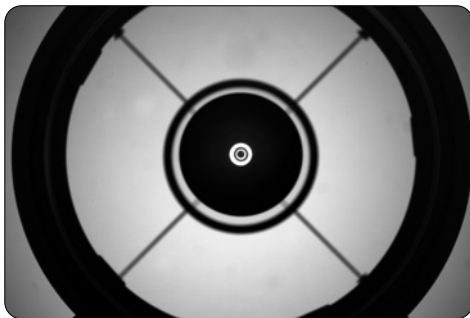
RC-Teleskop mit korrekt eingestelltem Sekundärspiegel, aber leicht dejustiertem Hauptspiegel; Colliscope auf Mittenmarkierung scharfgestellt.
