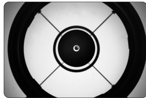
Dejustiertes RC-Teleskop
