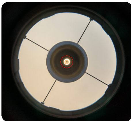
Dejustiertes RC-Teleskop
