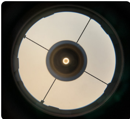
RC-Teleskop mit korrekt eingestelltem Sekundärspiegel, aber dejustiertem Hauptspiegel; Colliscope auf Fangpiegelspinne scharfgestellt.
