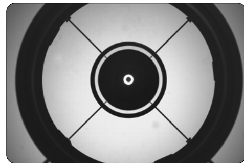
Justiertes RC-Teleskop, Colliscope auf Fangspiegelhalter scharfgestellt.
